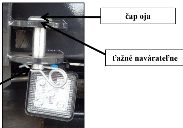
svetlo biele pozičné LED
