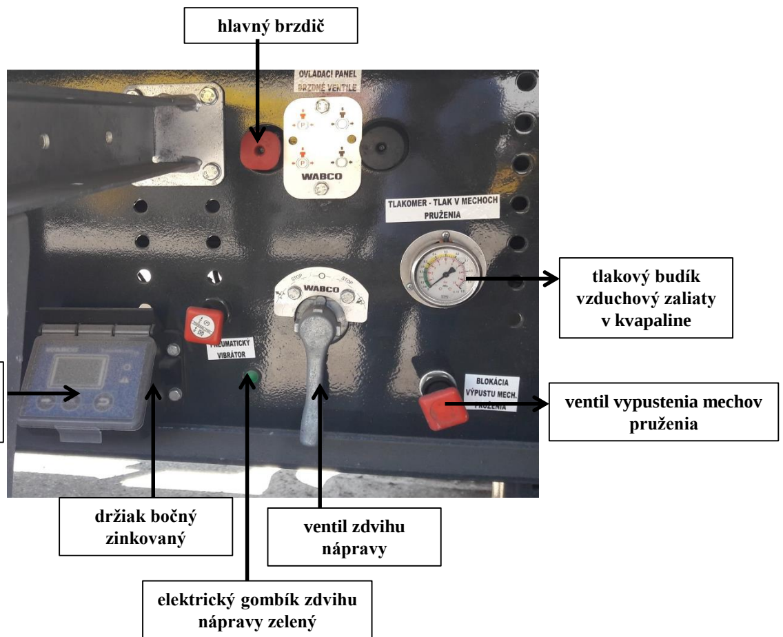
ventil odistenia zadnej poistky pneumatický
